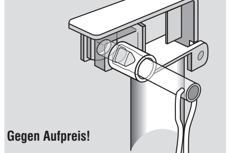
VERSCHLUSS C
