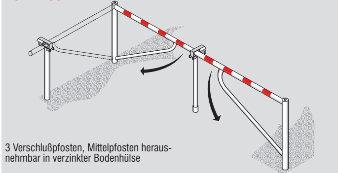
DOPPELSCHRANKE 7–12 m
