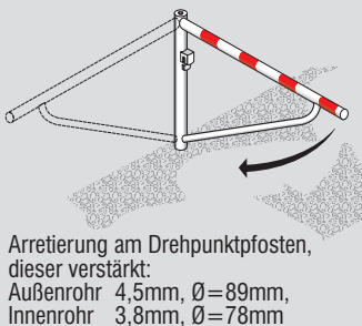
VERSCHLUSS A
